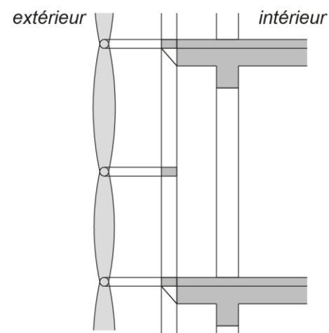
coupe
