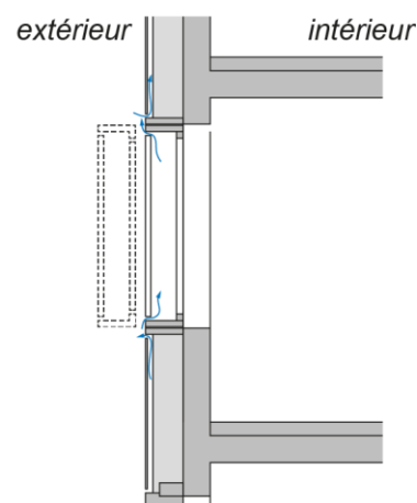
coupe
