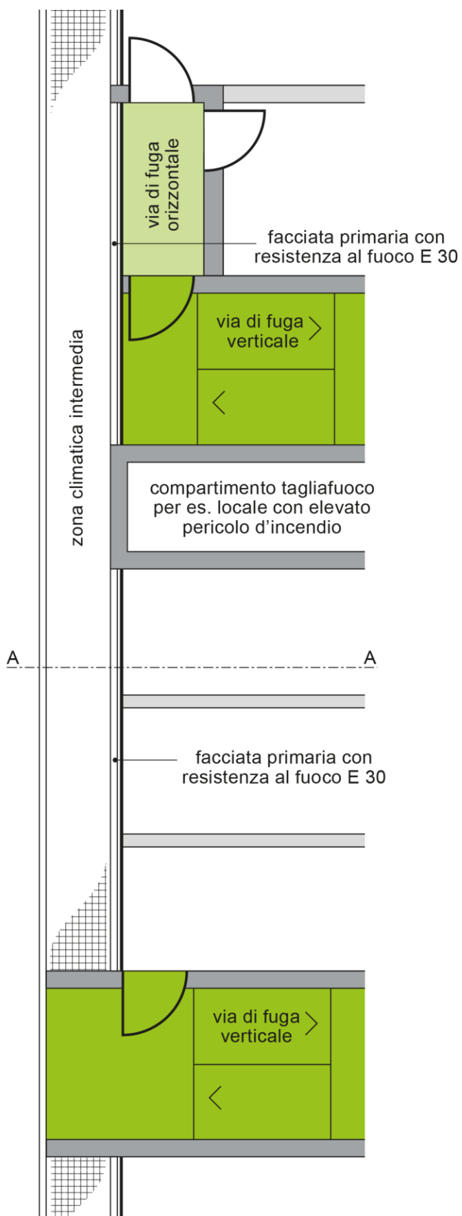
Pianta
