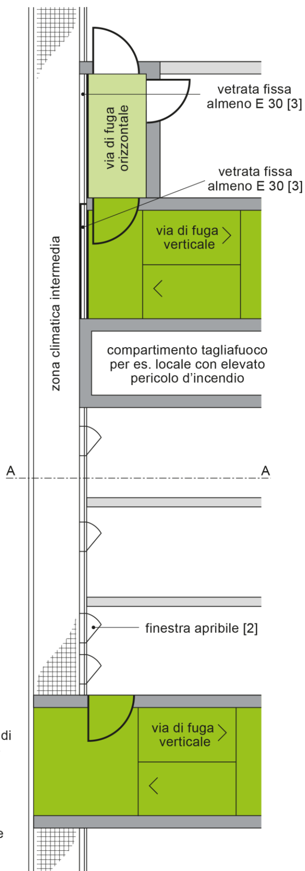
Pianta
